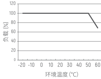
降额曲线
