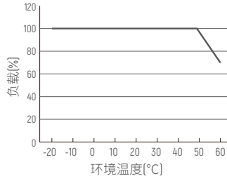
降额曲线
