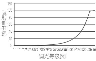
调光曲线
